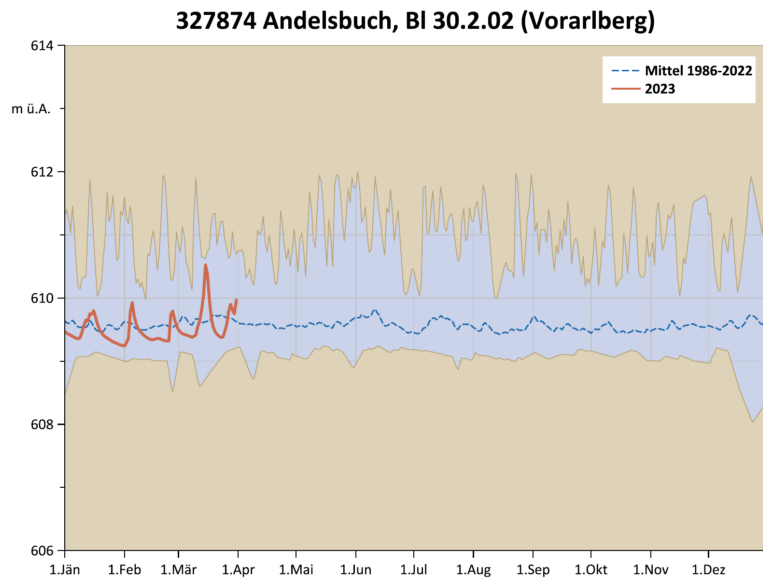
Abbildung 26. Tagesmittel des Grundwasserstandes 2023 (Rheintal, Bregenzer Wald, Montafon) im Vergleich zum langjährigen Tagesmittel und den Minima und Maxima der Tagesmittel des Vergleichszeitraums.
