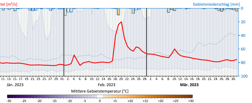
Abbildung 15. Pegel Lilienfeld-Markt und Zwettl. Obere Reihe: Abflussganglinien (Tagesmittel) 2023, langjährige Tagesmittelwerte sowie Minima und Maxima der Tagesmittel des Vergleichszeitraums. Untere Reihe: vergangene drei Monate mit zusätzlich dargestellten Tagesgebietsniederschlagssummen (Balken) und mittleren täglichen Gebietstemperaturen (Einfärbung Balken) in den Pegelinzugsgebieten.
