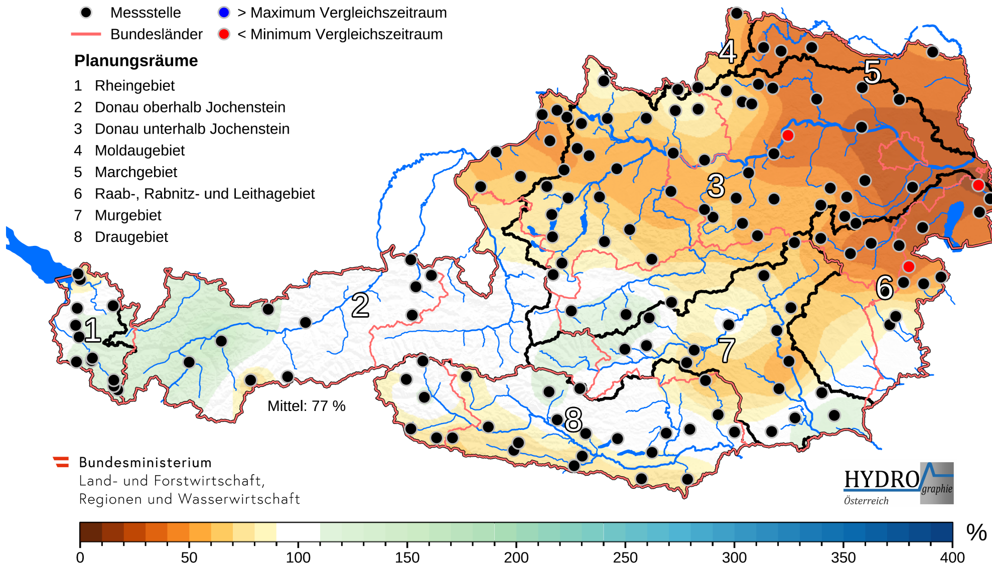
Abbildung 3. Niederschlagssumme des März 2023, ausgedrückt in Prozent der mittleren Niederschlagssumme im März im Vergleichszeitraum 1981-2010. Blau markierte Messstellen: Monatssumme des Niederschlags über der im Vergleichszeitraum aufgetretenen höchsten Monatssumme. Rot markierte Messstellen: Monatssumme des Niederschlags unter der im Vergleichszeitraum aufgetretenen niedrigsten Monatssumme.
