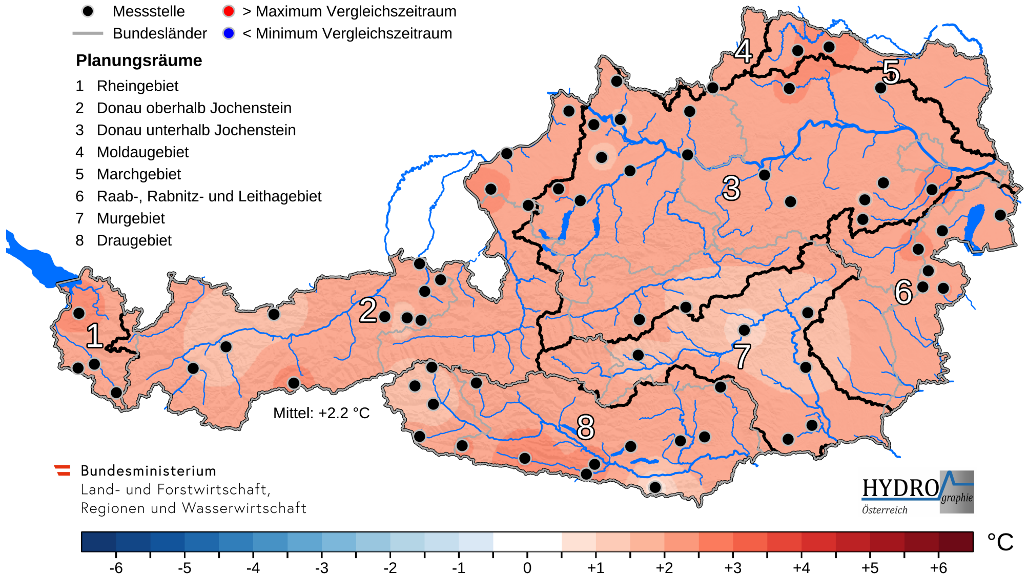
Abbildung 2. Temperaturabweichung in °C des März 2023 vom langjährigen Monatsmittel des Vergleichszeitraums 1981-2010. Rot markierte Messstellen: mittlere Monatstemperatur über dem im Vergleichszeitraum aufgetretenen höchsten Monatsmittel. Blau markierte Messstellen: mittlere Monatstemperatur unter dem im Vergleichszeitraum aufgetretenen niedrigsten Monatsmittel.
