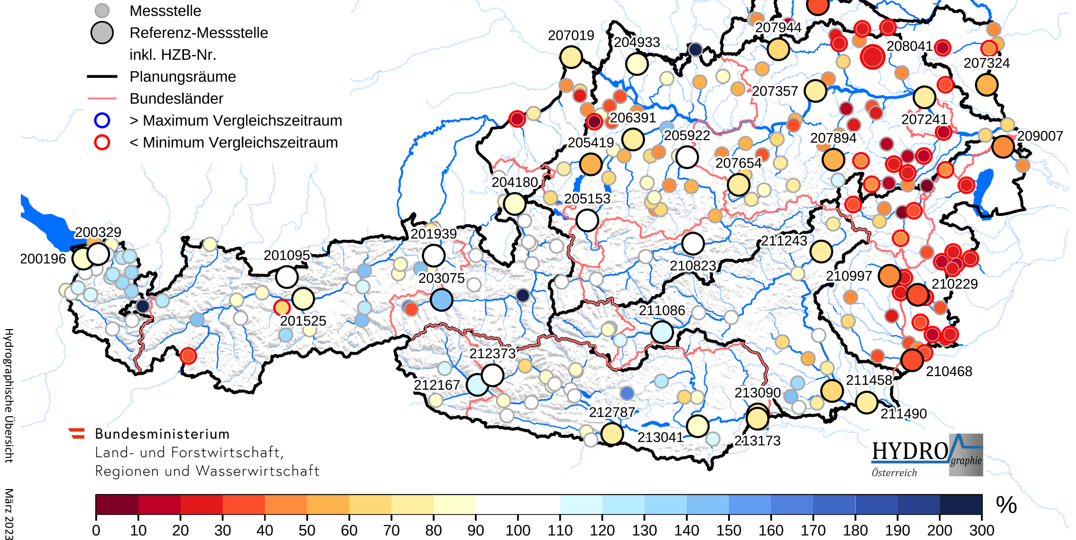
Abbildung 5. Mittlerer Monatsabfluss des März 2023, ausgedrückt in Prozent des langjährigen mittleren Abflusses im März. Ein Wert von 100 entspricht dem langjährigen Monatsmittel. Blau markierte Messstellen: mittlerer Monatsabfluss über dem im Vergleichszeitraum aufgetretenen Maximum. Rot markierte Messstellen: mittlerer Monatsabfluss unter dem im Vergleichszeitraum aufgetretenen Minimum. Der Vergleichszeitraum zur Ermittlung des langjährigen Mittels variiert an den Messstellen (mindestens zehn Jahre).
