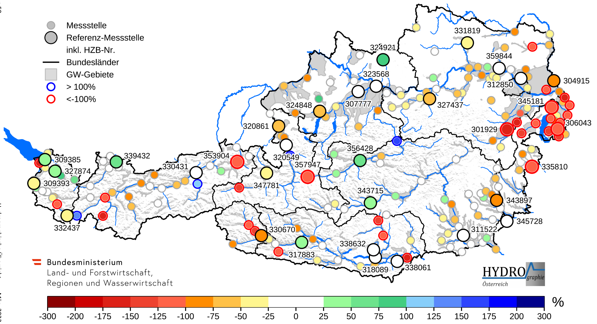
Abbildung 6. Grundwasserstand am letzten Tag des März 2023 im Vergleich zum langjährigen Mittelwert des letzten Tages im März. Ein Wert von 0 entspricht dem langjährigen Mittel, Werte zwischen -100 und 100 entsprechen der im Vergleichszeitraum aufgetretenen Schwankungsbreite. Werte > 100 und < -100 zeigen neue Extrema im negativen und positiven Bereich (zusätzlich blau und rot markiert). Der Vergleichszeitraum zur Ermittlung des langjährigen Mittels variiert an den Messstellen (mindestens zehn Jahre).
