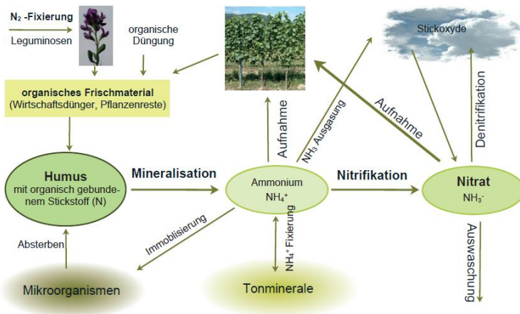
Abbildung 657: Stickstoffkreislauf
