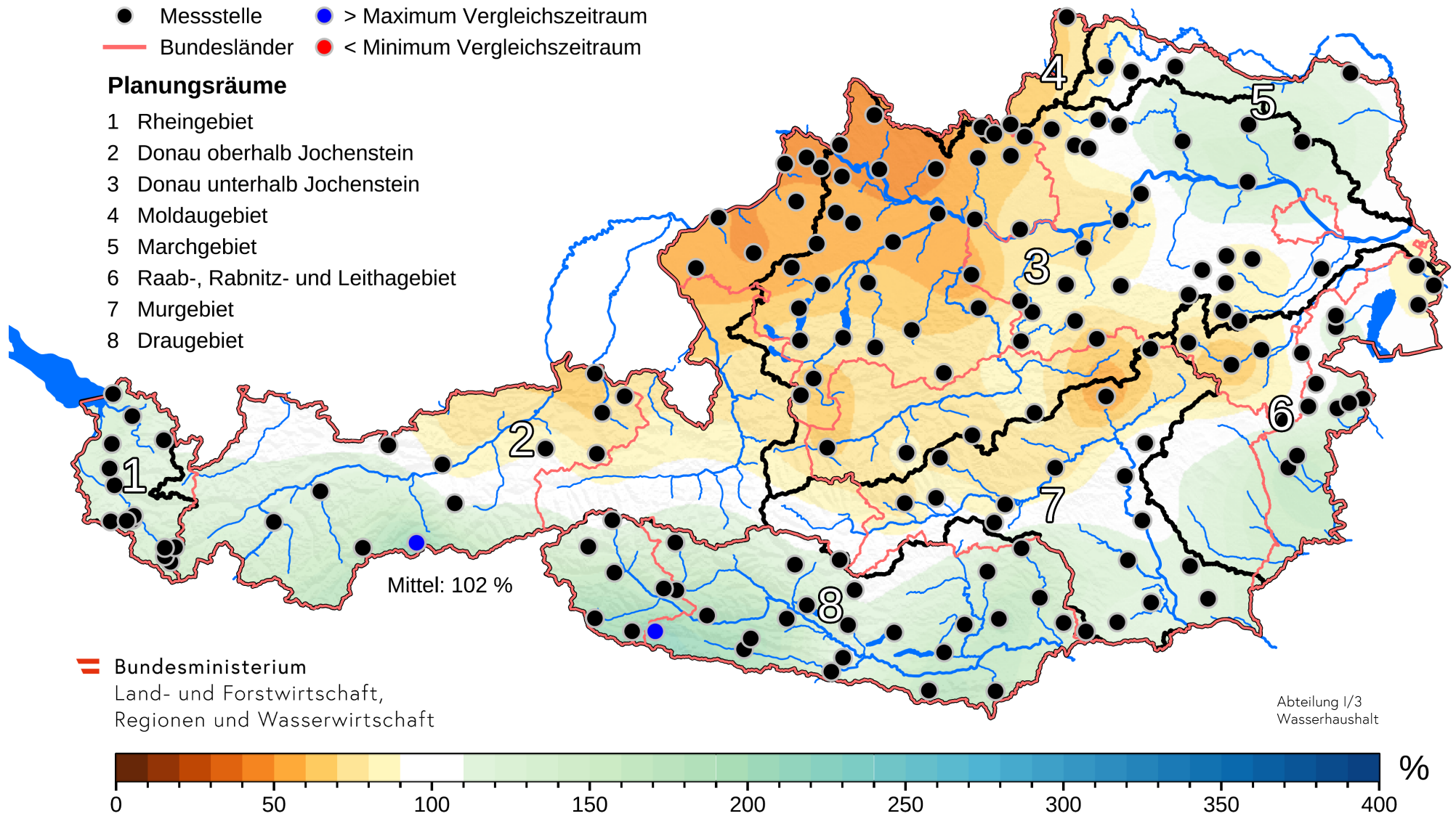
Abbildung 3. Niederschlagssumme des März 2024, ausgedrückt in Prozent der mittleren Niederschlagssumme im März im Vergleichszeitraum 1991-2020. Blau markierte Messstellen: Monatssumme des Niederschlags über der im Vergleichszeitraum aufgetretenen höchsten Monatssumme. Rot markierte Messstellen: Monatssumme des Niederschlags unter der im Vergleichszeitraum aufgetretenen niedrigsten Monatssumme.
