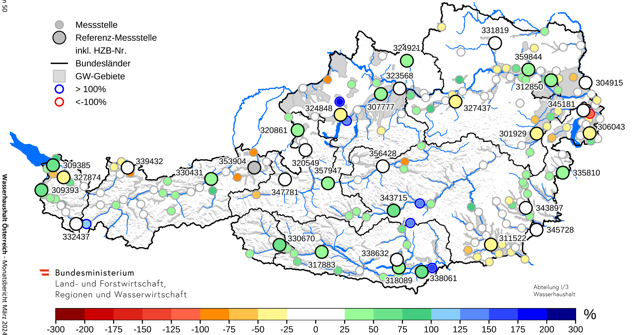
Abbildung 6. Grundwasserstand am letzten Tag des März 2024 im Vergleich zum langjährigen Mittelwert des letzten Tages im März. Ein Wert von 0 entspricht dem langjährigen Mittel, Werte zwischen -100 und 100 entsprechen der im Vergleichszeitraum aufgetretenen Schwankungsbreite, Werte > 100 und < -100 zeigen neue Extrema im negativen und positiven Bereich (zusätzlich blau und rot markiert). Der Vergleichszeitraum zur Ermittlung des langjährigen Mittels variiert an den Messstellen (mindestens zehn Jahre).
