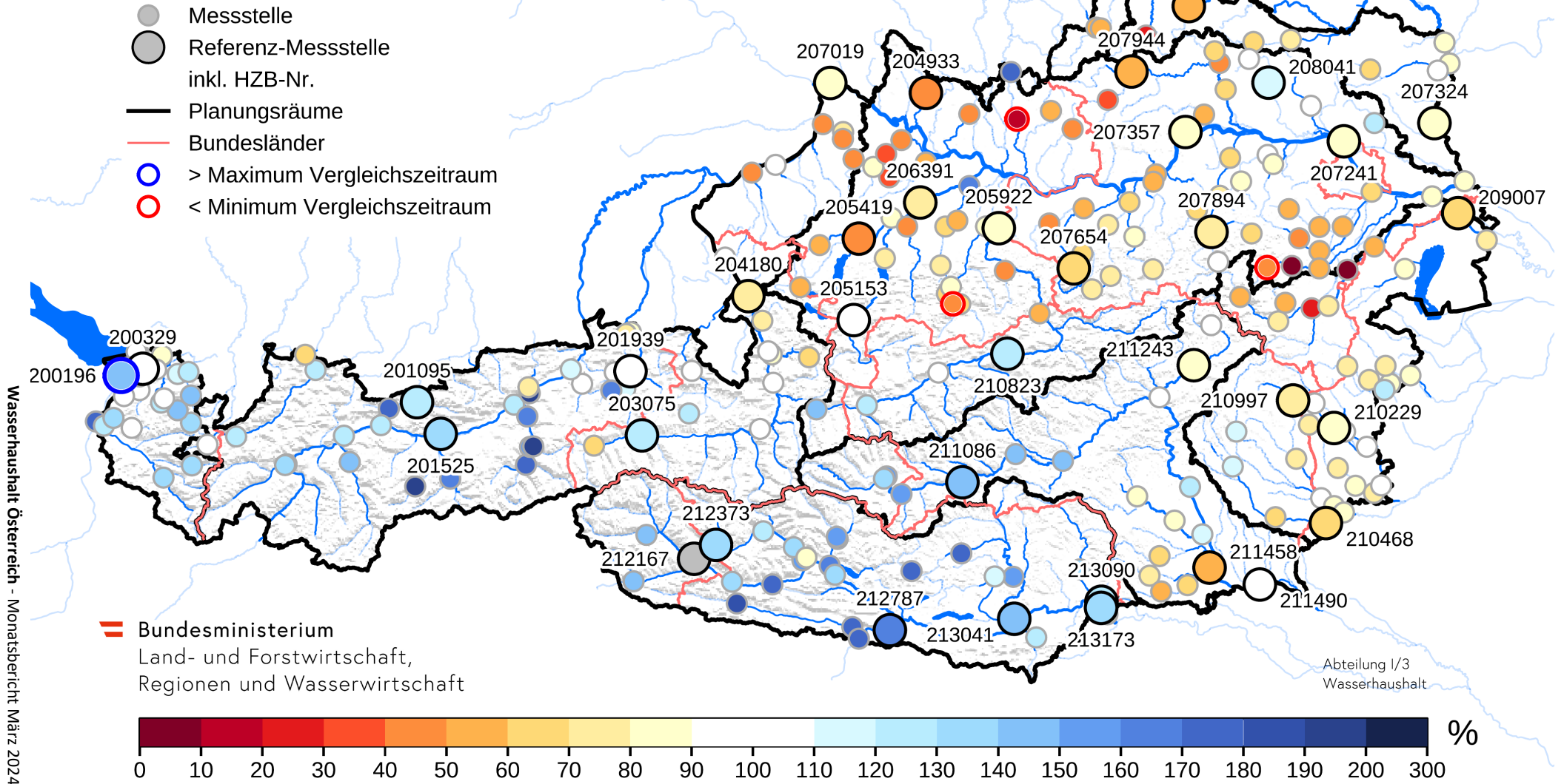
Abbildung 5. Mittlerer Monatsabfluss des März 2024, ausgedrückt in Prozent des langjährigen mittleren Abflusses im März, Ein Wert von 100 entspricht dem langjährigen Monatsmittel, Blau markierte Messstellen: mittlerer Monatsabfluss über dem im Vergleichszeitraum aufgetretenen Maximum, Rot markierte Messstellen: mittlerer Monatsabfluss unter dem im Vergleichszeitraum aufgetretenen Minimum, Vergleichszeitraum an den Messstellen: mindestens zehn Jahre der Periode 1991-2020.
