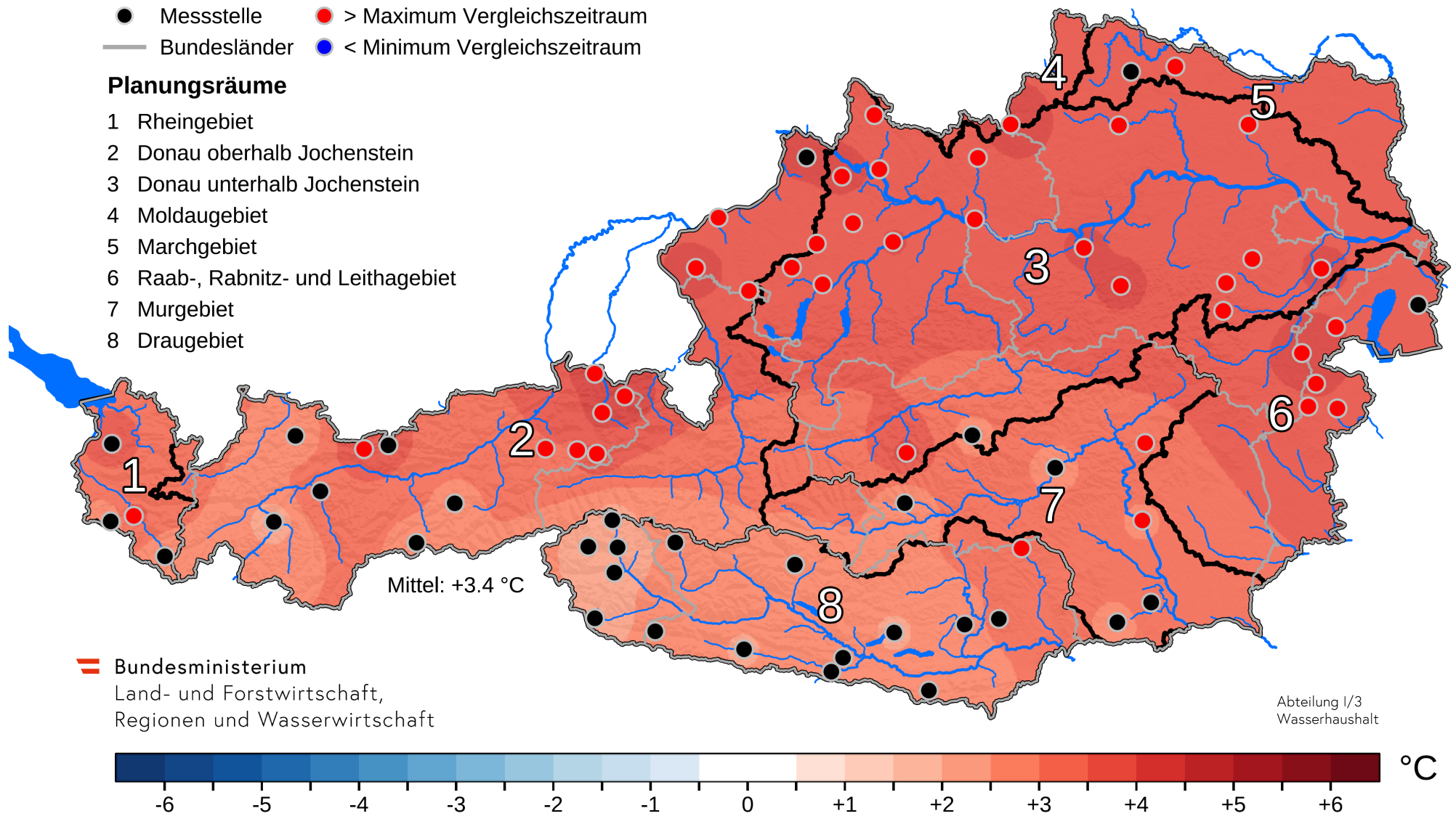
Abbildung 2. Temperaturabweichung in °C des März 2024 vom langjährigen Monatsmittel des Vergleichszeitraums 1991-2020. Rot markierte Messstellen: mittlere Monatstemperatur über dem im Vergleichszeitraum aufgetretenen höchsten Monatsmittel. Blau markierte Messstellen: mittlere Monatstemperatur unter dem im Vergleichszeitraum aufgetretenen niedrigsten Monatsmittel.
