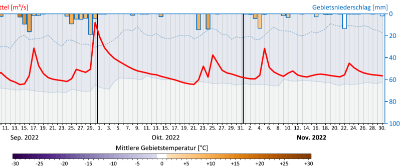
Abbildung 23. Pegel Federaun und Gumisch. Obere Reihe: Abflussganglinien (Tagesmittel) 2022, langjährige Tagesmittelwerte sowie Minima und Maxima der Tagesmittel des Vergleichszeitraums. Untere Reihe: vergangene drei Monate mit zusätzlich dargestellten Tagesgebietsniederschlagssummen (Balken) und mittleren täglichen Gebietstemperaturen (Einfärbung Balken) in den Pegelinzugsgebieten.
