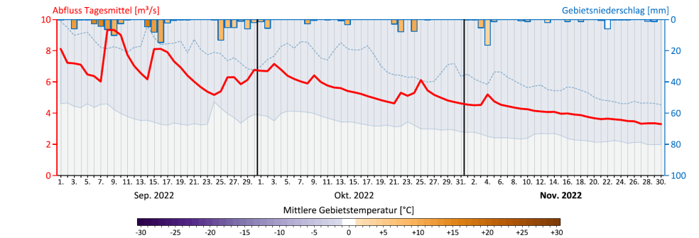
Abbildung 22. Pegel Lienz und Winklern. Obere Reihe: Abflussganglinien (Tagesmittel) 2022, langjährige Tagesmittelwerte sowie Minima und Maxima der Tagesmittel des Vergleichszeitraums. Untere Reihe: vergangene drei Monate mit zusätzlich dargestellten Tagesgebietsniederschlagssummen (Balken) und mittleren täglichen Gebietstemperaturen (Einfärbung Balken) in den Pegelinzugsgebieten.
