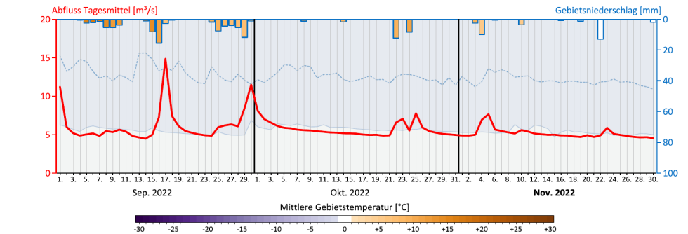
Abbildung 24. Pegel Lavamünd Ort und Krottendorf. Obere Reihe: Abflussganglinien (Tagesmittel) 2022, langjährige Tagesmittelwerte sowie Minima und Maxima der Tagesmittel des Vergleichszeitraums. Untere Reihe: vergangene drei Monate mit zusätzlich dargestellten Tagesgebietsniederschlagssummen (Balken) und mittleren täglichen Gebietstemperaturen (Einfärbung Balken) in den Pegelinzugsgebieten.
