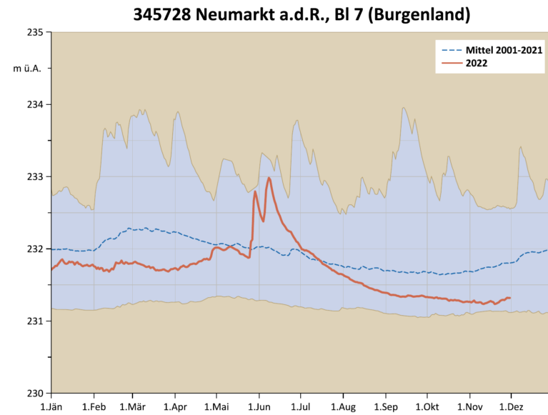
Abbildung 34. Tagesmittel des Grundwasserstandes 2022 (Parndorfer Platte, Seewinkel, Rabnitztal, Raabtal) im Vergleich zu langjährigen Tagesmittel, Minima und Maxima.
