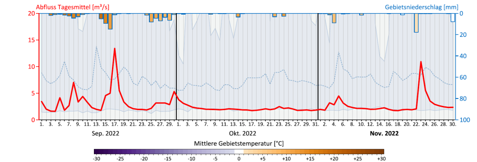
Abbildung 18. Pegel Deutsch Haslau und Neumarkt. Obere Reihe: Abflussganglinien (Tagesmittel) 2022, langjährige Tagesmittelwerte sowie Minima und Maxima der Tagesmittel des Vergleichszeitraums. Untere Reihe: vergangene drei Monate mit zusätzlich dargestellten Tagesgebietsniederschlagssummen (Balken) und mittleren täglichen Gebietstemperaturen (Einfärbung Balken) in den Pegelinzugsgebieten.
