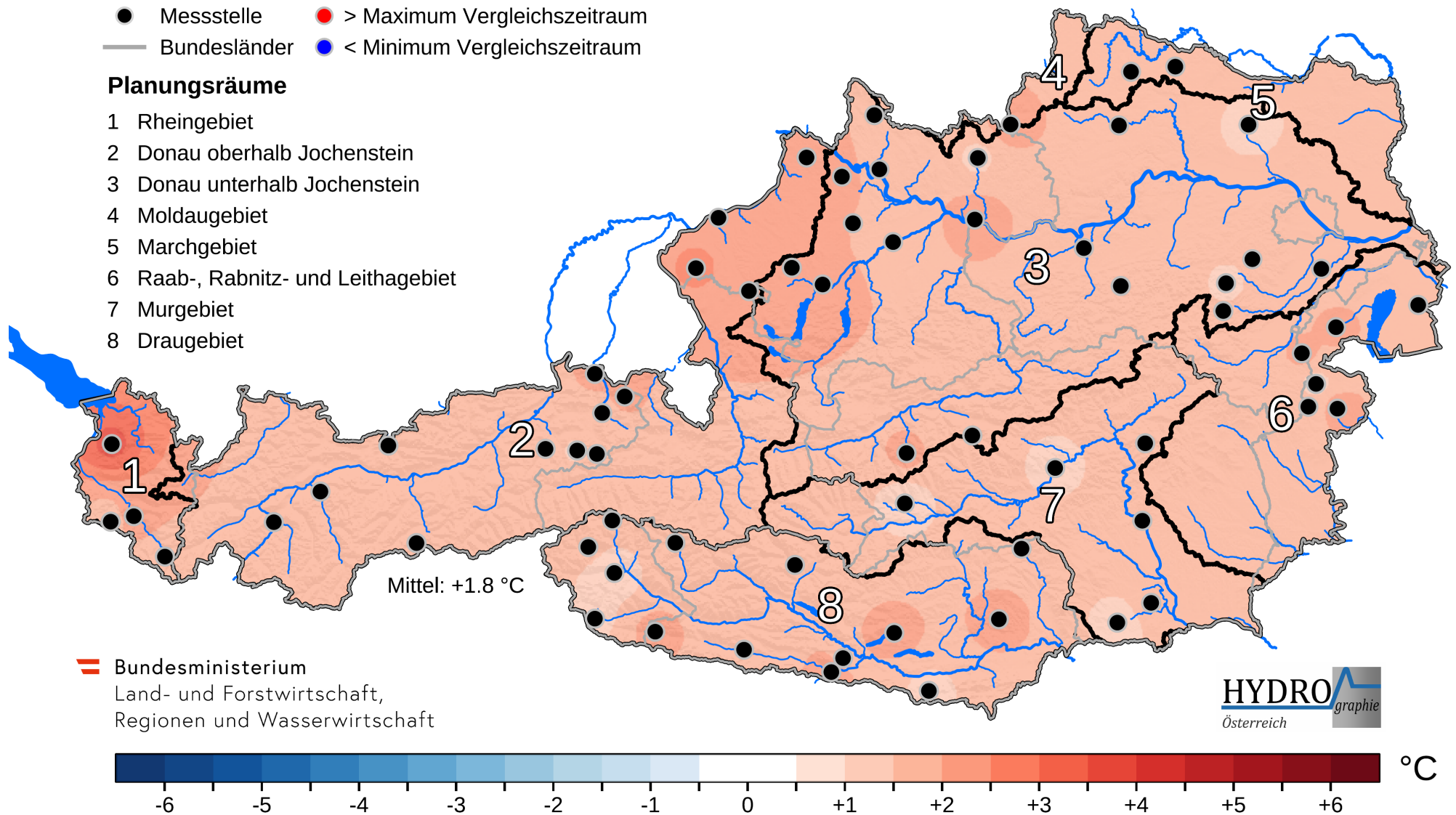
Abbildung 2. Temperaturabweichung in °C des November 2022 vom langjährigen Monatsmittel des Vergleichszeitraums 1981-2010. Rot markierte Messstellen: mittlere Monatstemperatur über dem im Vergleichszeitraum aufgetretenen höchsten Monatsmittel. Blau markierte Messstellen: mittlere Monatstemperatur unter dem im Vergleichszeitraum aufgetretenen niedrigsten Monatsmittel.
