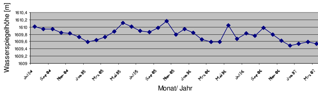
Wasserstand im Piezometerstandrohr
