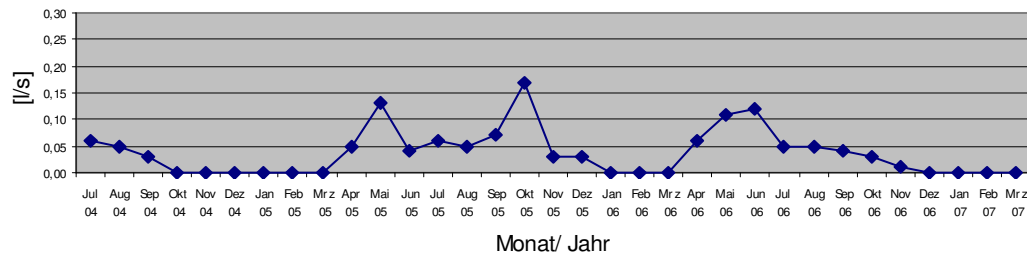
Sickerwasserverlauf Summe 1-3
