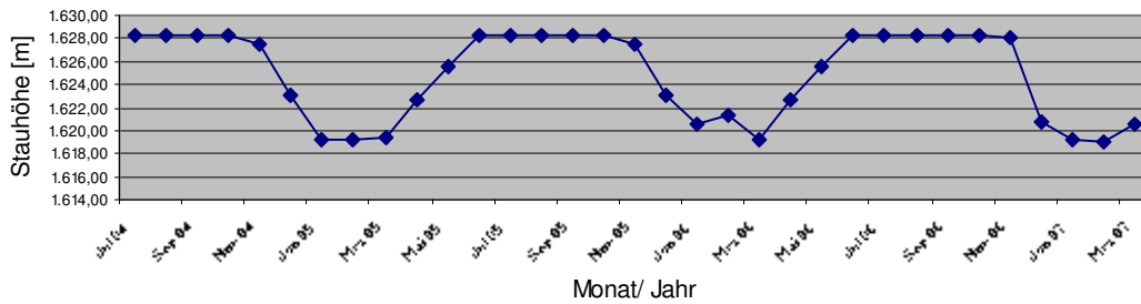
Verlauf der Staulinie
