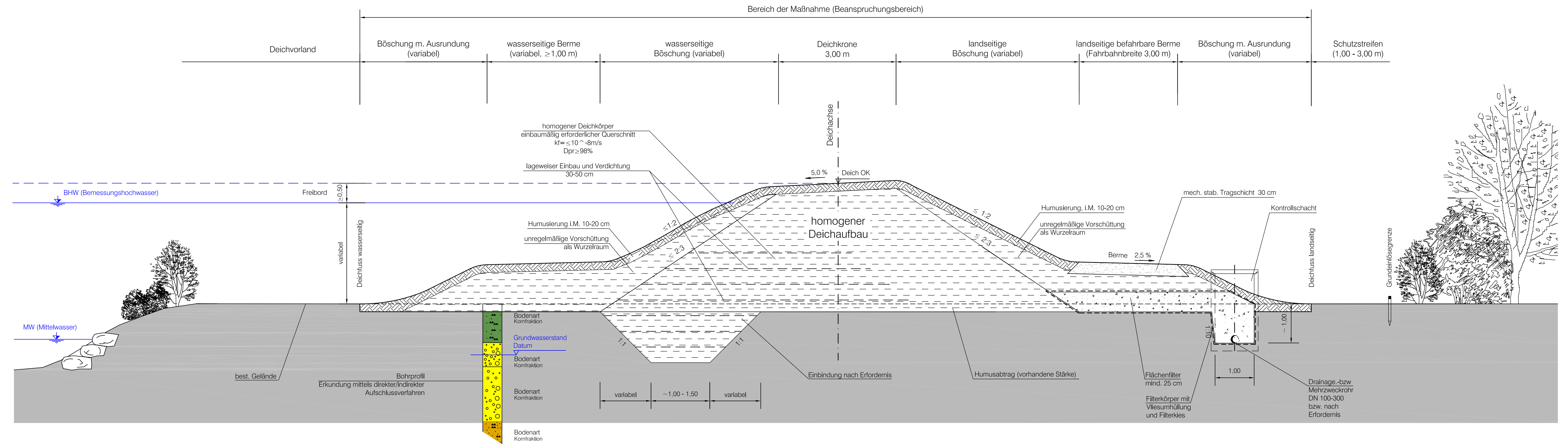
Musterdeich Mindestquerschnitt Homogendeich, beidseitige Bermen (optional)
